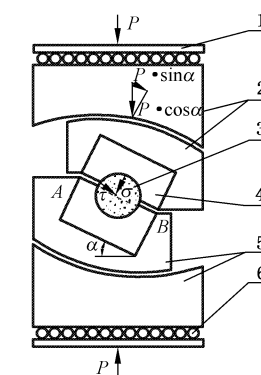
1——钢垫板; 2——变角剪切夹具上座; 3——标准试件; 4——圆柱体标准试件剪切模具; 5——变角剪切夹具下座; 6——滚柱。
